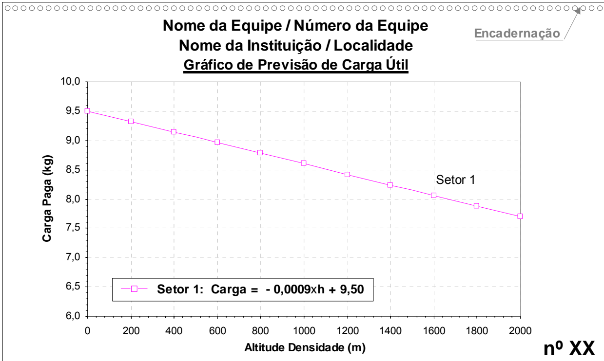
Figura acima: Exemplo de Gráfico para Classe Regular para o Setor 1 somente. Ver seção 5.1.4.1. Encadernar conforme indicação na figura acima. O gráfico deve ser em Landscape.
