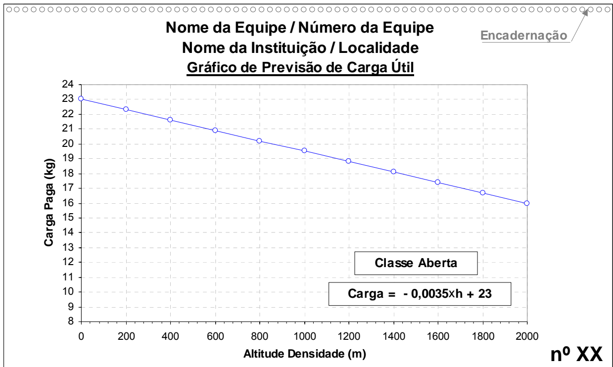
Figura acima: Exemplo de Gráfico para Classe Aberta. Ver seção 5.1.4.1. Para a Classe Aberta a decolagem segmentada não é válida. Será usada a pista normal ou 61m. Encadernar conforme indicação na figura acima. O gráfico deve ser em Landscape.
